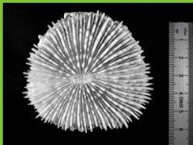
Taxonomie corallienne
