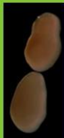
Etude de la ponte, du recrutement et de la croissance des coraux
